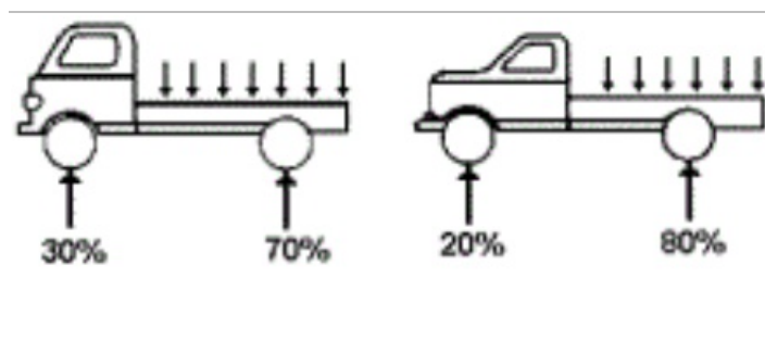
平头卡车
