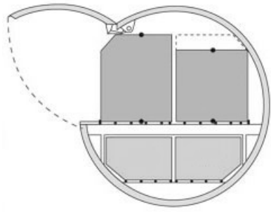
侧装货舱
